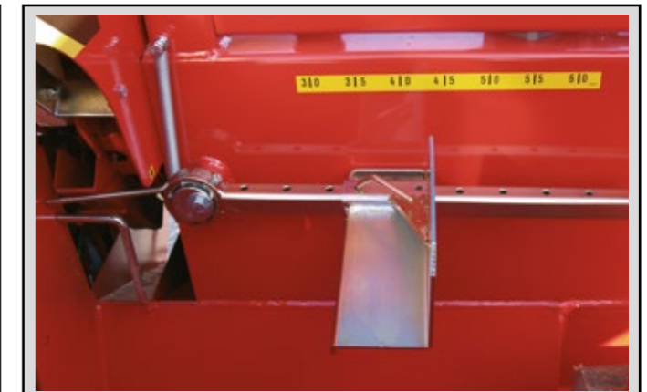
Excenter den Längsanschlag minimal vom Holz weg und ermöglicht den freien Fall in den Spaltkanal.
