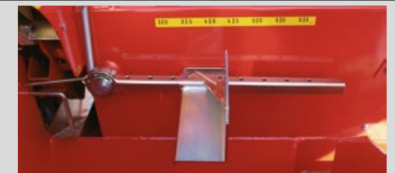
Excenter - Beim Sägevorgang bewegt ein mech. Excenter den Längsanschlag minimal vom Holz weg und ermöglicht den freien Fall in den Spaltkanal.
